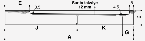
Kesit A-A
