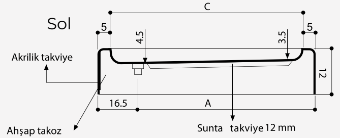
Kesit A-A
