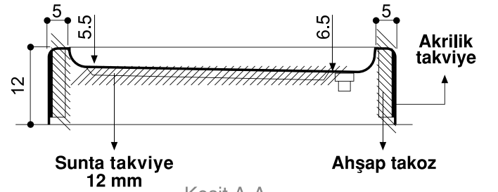
Kesit A-A
