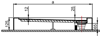
Kesit A-A
