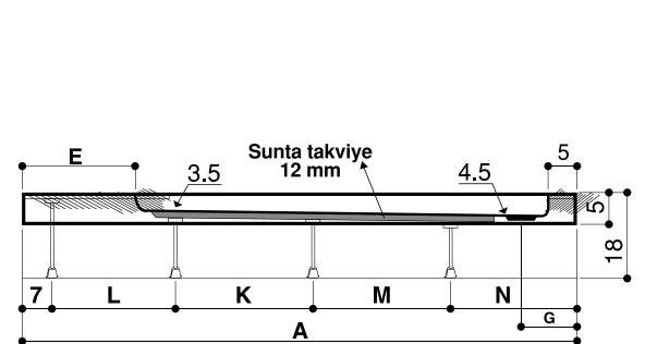
Kesit A-A
