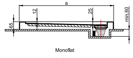
Kesit A-A
