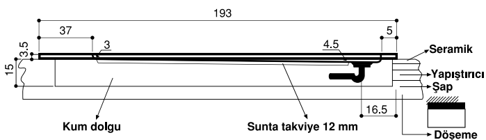
Kesit A-A
