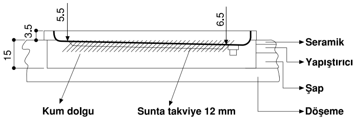
Kesit A-A
