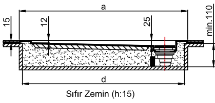
Kesit A-A
