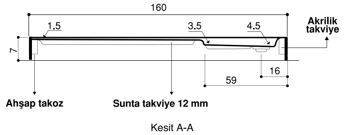
Kesit A-A
