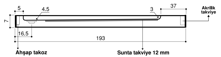
Kesit A-A
