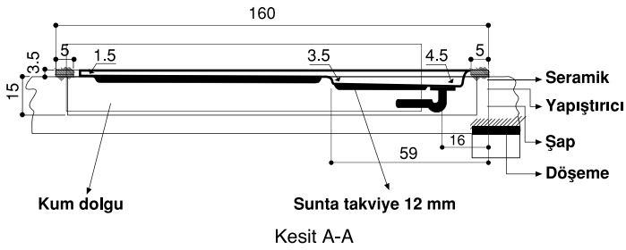
Kesit A-A
