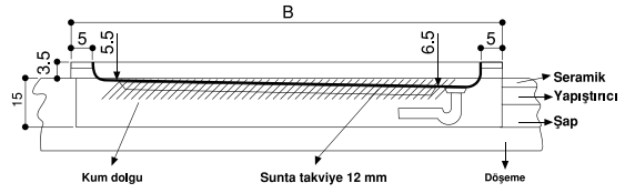
Kesit A-A
