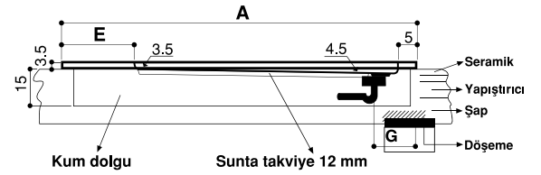
Kesit A-A
