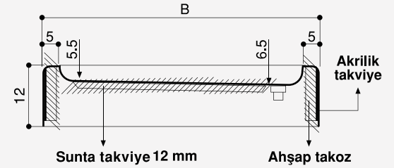
Kesit A-A
