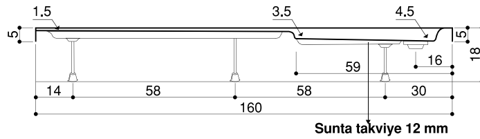
Kesit A-A
