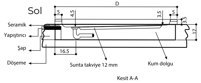
Kesit A-A
