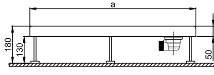
Kesit A-A
