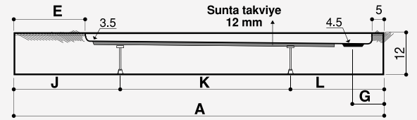
Kesit A-A
