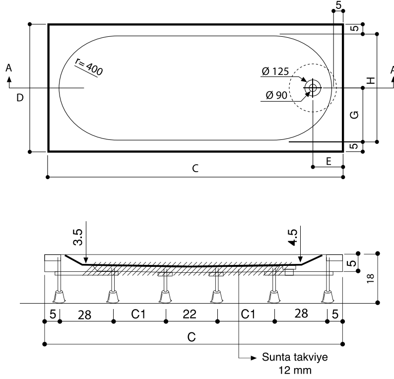
Kesit A-A
